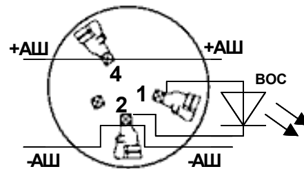
Рис. 1. Подключение базового основания В401 к адресной шине и к ВОС
