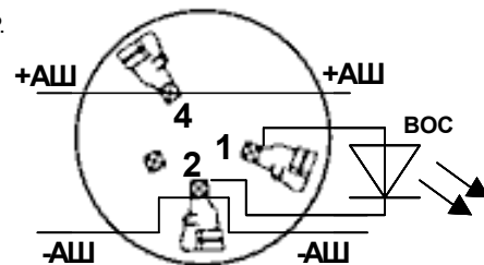
Рис. 1. Подключение базового основания серии В401L к адресной шине и к ВОС
